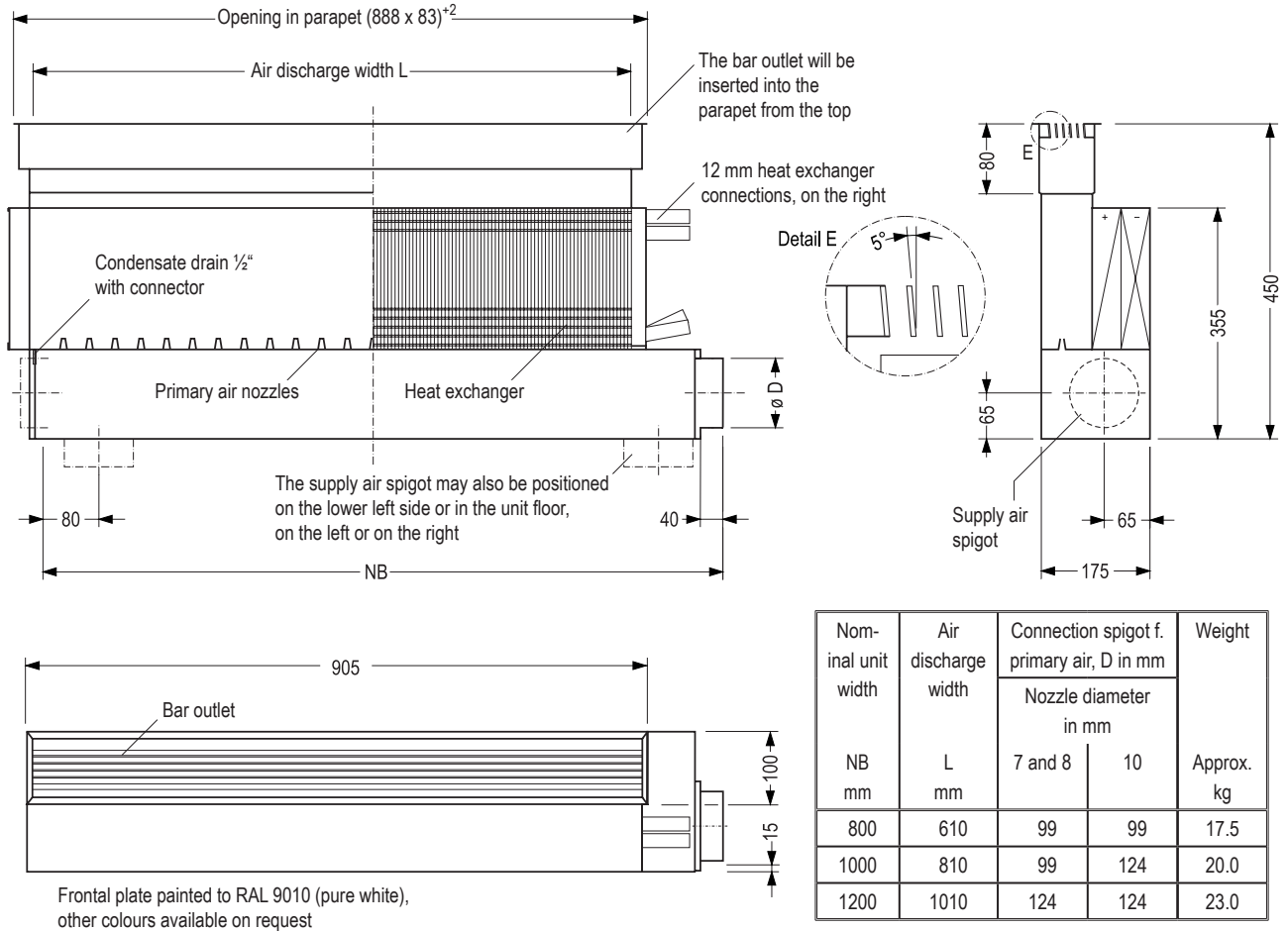
Fig. 3: Unit dimensions
